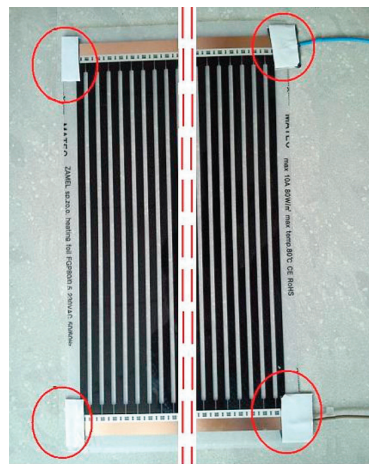
Abb. 2. Stellen die mit Isoliertape isoliert werden müssen, um vor Stromschlag zu schützen.
