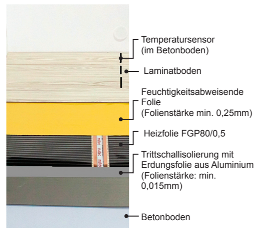
Abb. 3. Schichtaufbau
