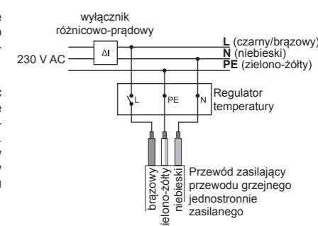
Rys. Schemat podłączenia przewodu grzejnego za pośrednictwem regulatora temperatury do instalacji elektrycznej.
