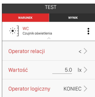
Przykładowy warunek dla czujnika natężenia oświetlenia
