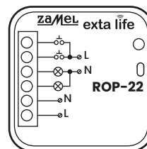
RADIOWY ODBIORNIK DOPUSZKOWY 2-KANAŁOWY ROP-22
