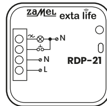
RADIOWY ŚCIEMNIACZ OŚWIETLENIA RDP-21
