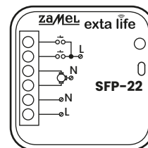
RADIOWY STEROWNIK ŻALUZJI FASADOWYCH SFP-22
