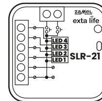
STEROWNIK LED 4-KANAŁOWY SLR-21
