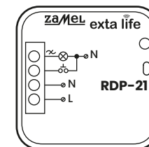
RADIOWY ŚCIEMIACZ OŚWIETLENIA RDP-21
