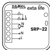
RADIOWY STEROWNIK ROLET DOPUSZKOWY SRP-22
