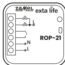
RADIOWY ODBIORNIK DOPUSZKOWY 1-KANAŁOWY ROP-21
