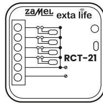
CZUJNIK TEMPERATURY DOPUSZKOWY RCT-21
