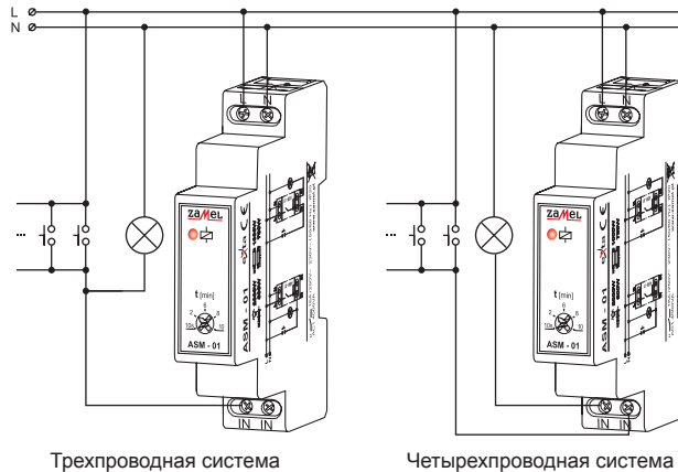
Трехпроводная система
