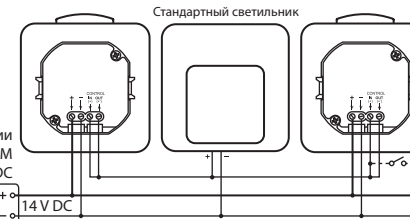
Блок питания серии ZNP, ZNN или ZNM версия 14 V DC
